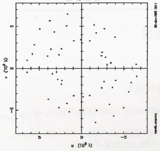
Capella (Oct 1997, 238.36T THz) AD1 AD2 AD3 AD4
